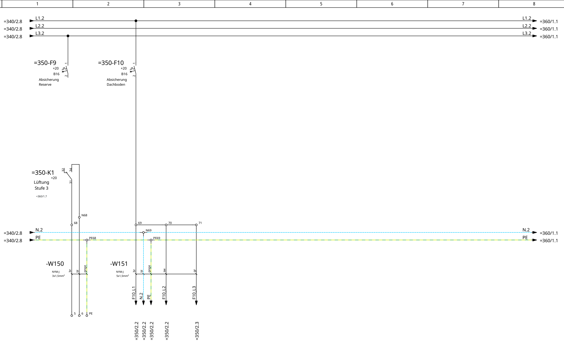
Klemmkasten Lüftungsanlage
